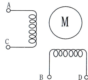
电气原理图
